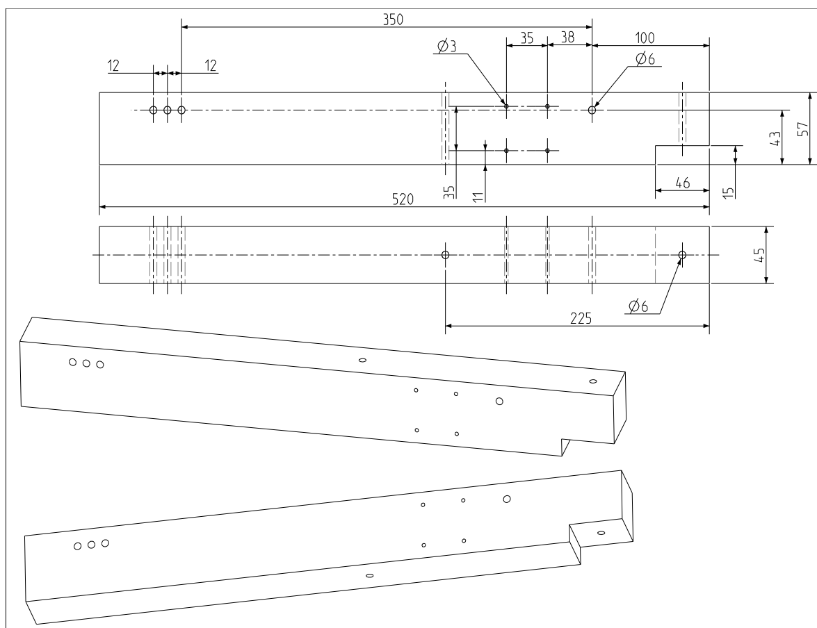
Figure 54 : Détail Longerons
