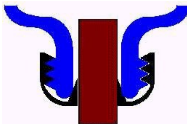
Figure 41 : Étanchéité à l'aide d'un bouchon à collerette
