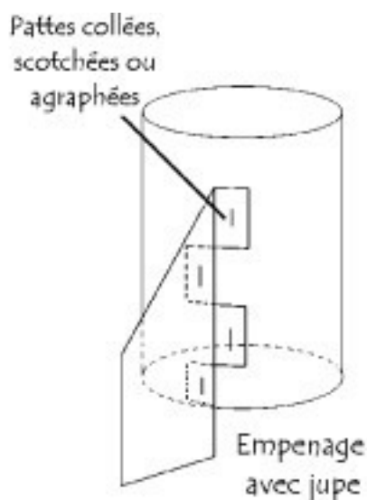
Figure 4 : fixation des ailerons sur la jupe
