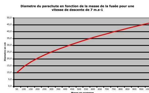
Figure 79 : Diamètre du parachute en fonction de la masse et d'une vitesse de descente de 7 \text{m.s}^{-1}
