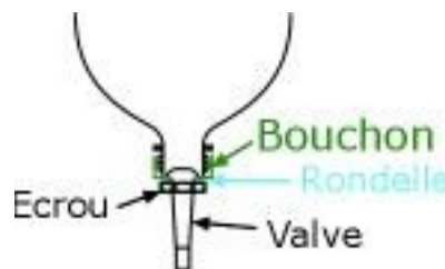
Figure 19 : Bouchon gonfleur
