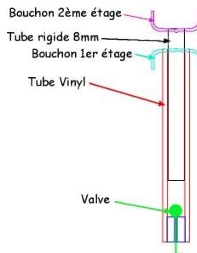
Figure 88 : Système de séparation d'une fusée multi-étages
