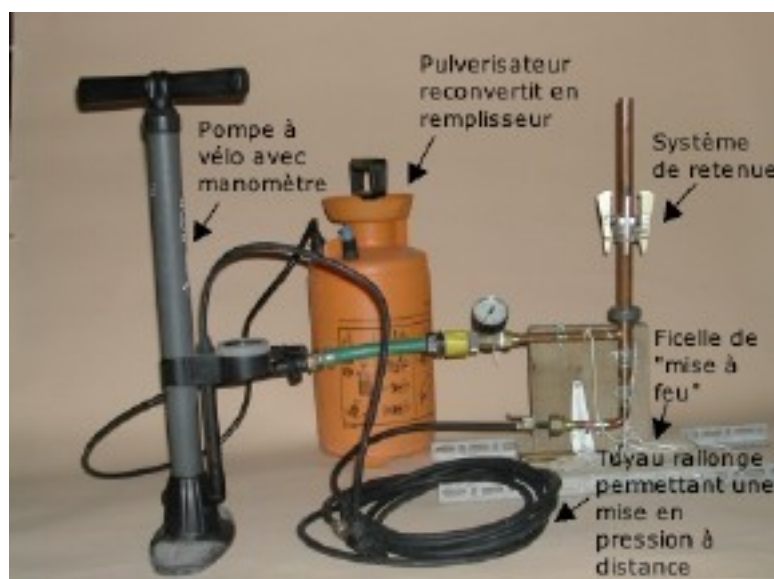
Figure 48 : Base de lancement complète avec lanceur, pompe à vélo, remplisseur d'eau
