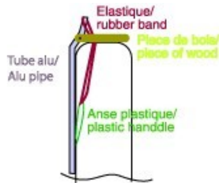
Figure 75 : Schéma explicatif de la photo ci-dessous, qui montre le système de déploiement des ailes
