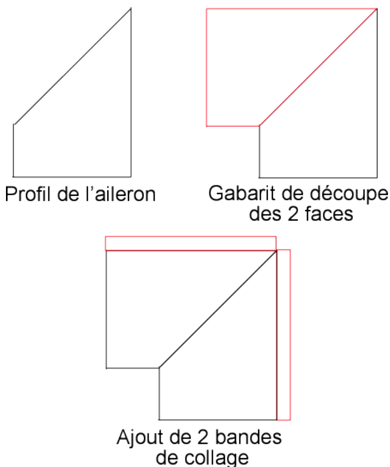
Figure 30 : Découpe d'un ailerons
